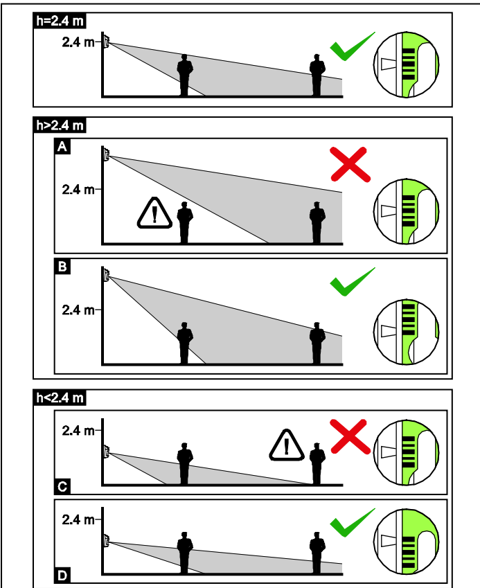
Рис. 7. Влияние высоты монтажа на охраняемую площадь и способ позиционирования пирозлемента по отношению к линзе с целью оптимальной установки. В зависимости от высоты монтажа средний штрих шкалы должен находиться напротив отметки на корпусе (монтаж на высоте 2,4 м), выше отметки (монтаж выше 2,4 м – см. В) или ниже отметки (монтаж ниже 2,4 м – см. D).
